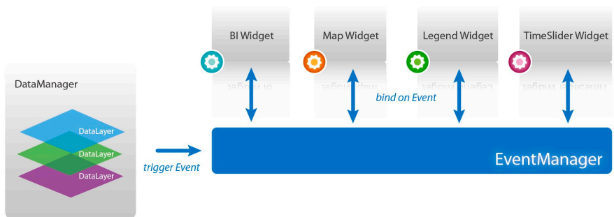
Abb. 3 Widget Architektur
